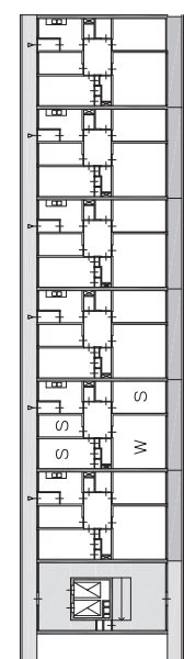
woonlaag, 1:500
